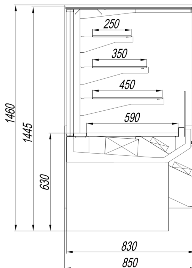
Рисунок 3. Внешний вид витрины ГРАНАТ КОМПАКТ КУБ 125 и ее сечение
