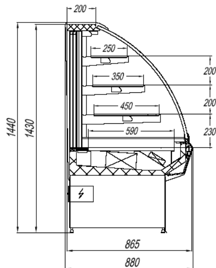
Рисунок 2. Внешний вид витрины ГРАНАТ КОМПАКТ 250 и ее сечение
