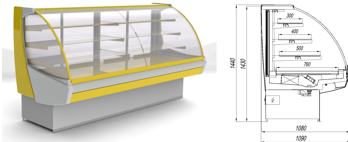
Рисунок 1. Внешний вид витрины ГРАНАТ 250 и ее сечение
