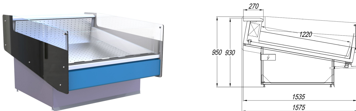
Рисунок 1. Внешний вид и сечение витрины «РЫБНЫЙ СТОЛ»
